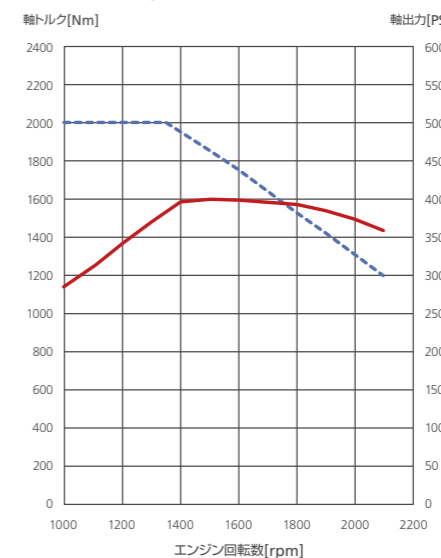
GH11TB2 400PS (ESCOT-VI) 294kW(400PS)/1,600rpm 2,000Nm(203kg·m)/1,200rpm
