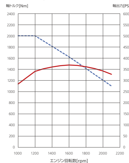
GH11TA2 370PS (ESCOT-VI) 272kW(370PS)/1,600rpm 2,000Nm(203kg·m)/1,200rpm
