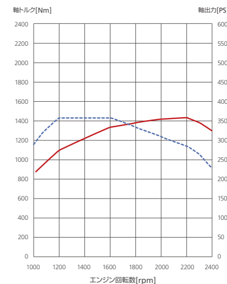
GH8TA 357PS (ESCOT-VI) 263kW(357PS) / 2,200rpm 1,428Nm(145.6kg·m) / 1,200-1,600rpm
